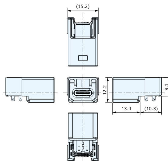
Receptacle : CSS5324-1R□□F
