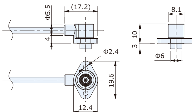
プラグ(ライトアングルタイプ)：CRS9001-3101F
