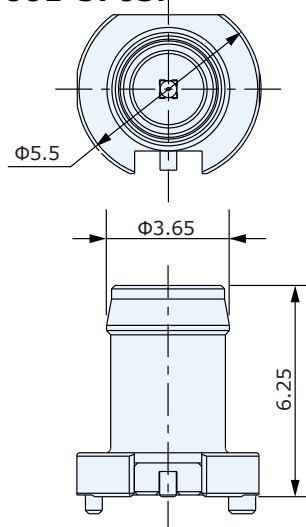
レセプタクル：CRC5001-8301F
