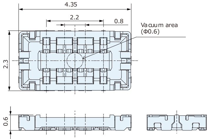
プラグ : CPBA306-0101F
