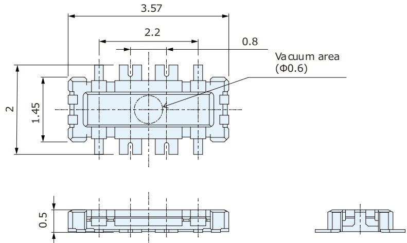
プラグ : CPBA306-0101F
