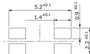
取付基板参考図
