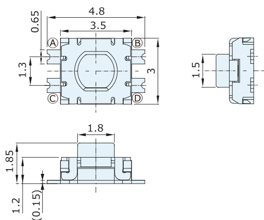
外形図
