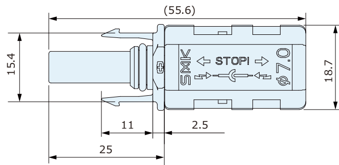
<插头 / 插座嵌合后>
