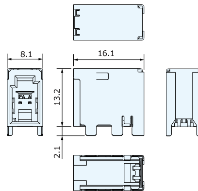
プラグ : CSC5002-3G□□F
