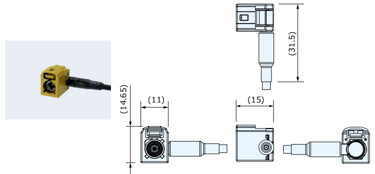
ケーブルジャック (低背・防水) CZF2100-03□□F
