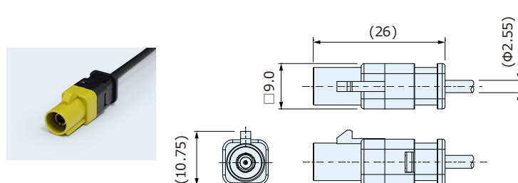
ケーブルプラグ (回転) CRC1001-56□□F
