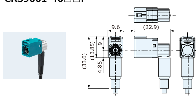
ケーブルジャック (防水) CRS9001-46□□F
