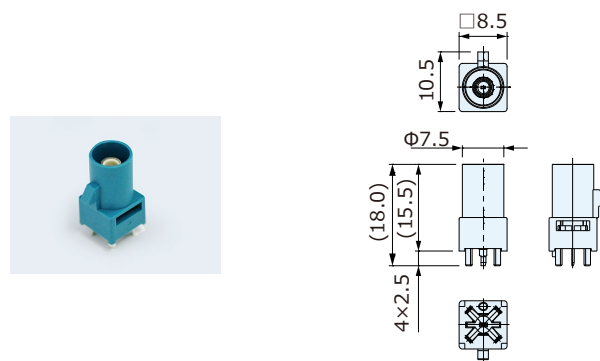
基板用プラグ CRC5001-64□□F
