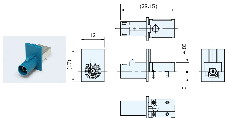
基板用プラグ(ミッドマウント・防水) CRC5001-74□□F
