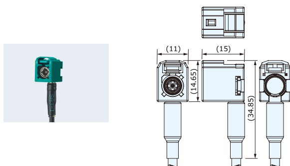
ケーブルジャック (低背・防水) CZF2100-13□□F
