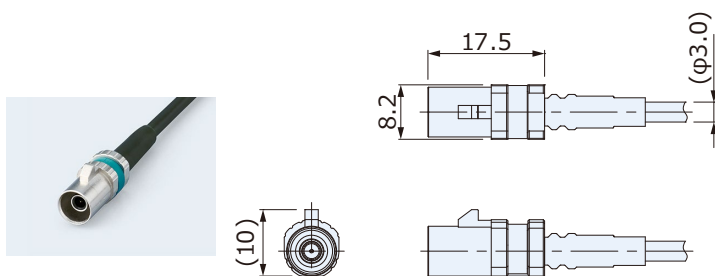
ケーブルプラグ (防水) CRC1001-57□□F
