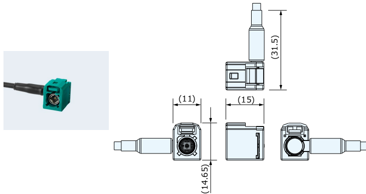
ケーブルジャック (低背・防水) CZF2100-02□□F
