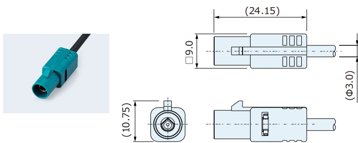
ケーブルプラグ CRC1001-52□□F
