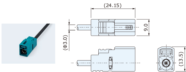
ケーブルジャック CRS9001-23□□F
