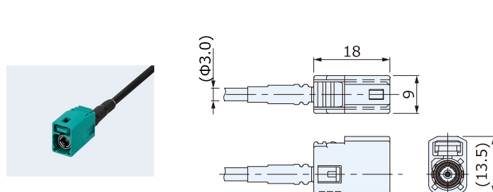
ケーブルジャック (防水) CRS9001-45□□F
