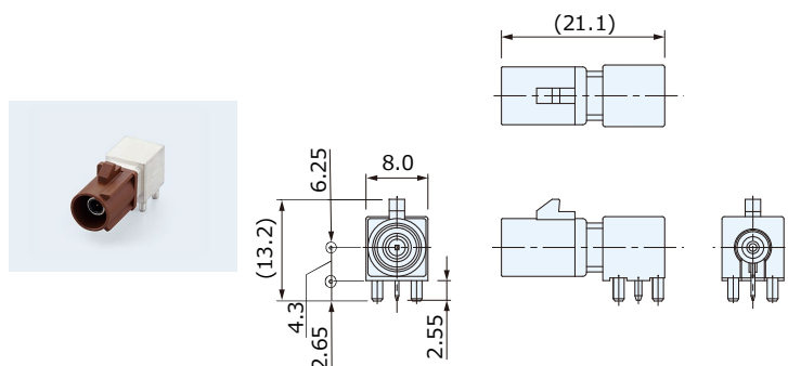
基板用プラグ CRC5001-70□□F
