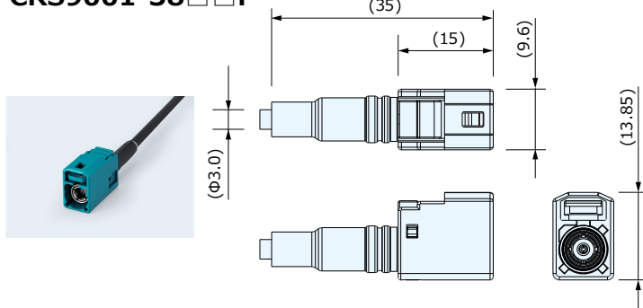
ケーブルジャック (防水・回転) CRS9001-38□□F
